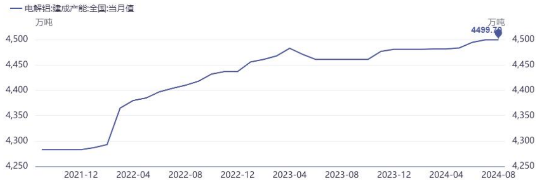
电解铝:建成产能:全国:当月值
