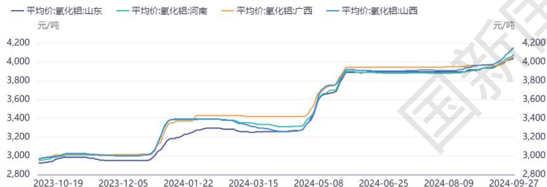
氧化铝:地区均价
