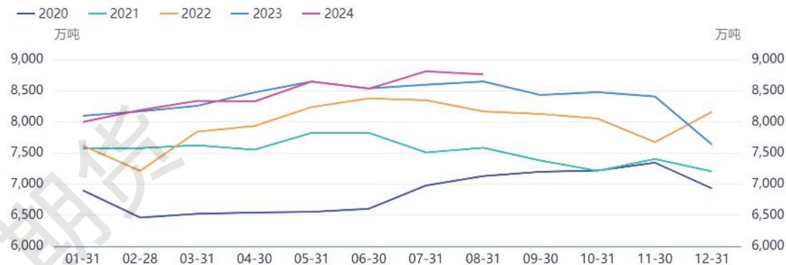
氧化铝:运行产能:全国:当月值
